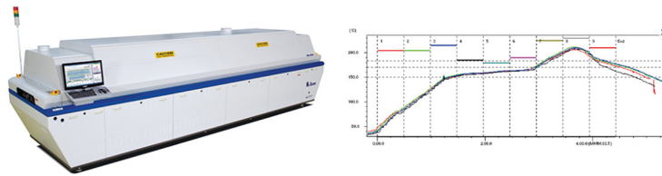
패키지 실장 평가 시스템(Reflow)
