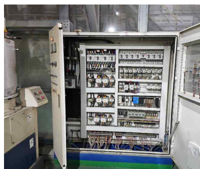
메인판넬 내부 전체 (메인 제어판넬 설치)
